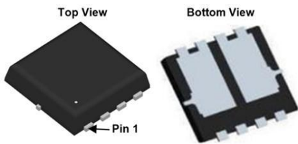
PDFN3x3-8L-D
